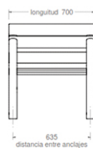
vista alzado 1:20
