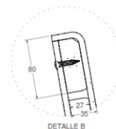
DETALLE B
