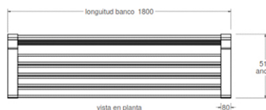
vista en planta 1:20
