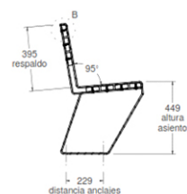
vista lateral 1:20
