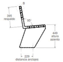
vista lateral 1:20
